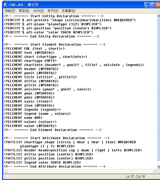
(그림 2) CML DTD
