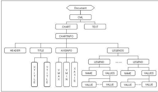
(그림 8) CML 문서에 대한 DOM 트리
