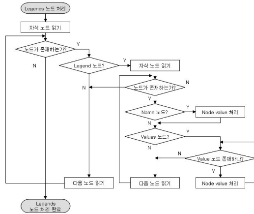
(그림 10) <Legends> 노드를 처리하기 위한 흐름도
