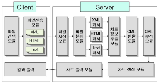
(그림 5) 차트출력시스템 구조도
