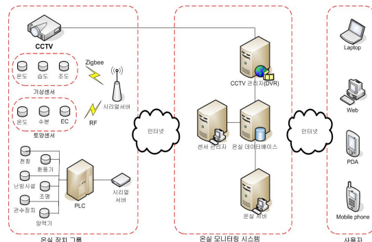
(그림 13) 유비쿼터스 온실관리시스템 구성도
