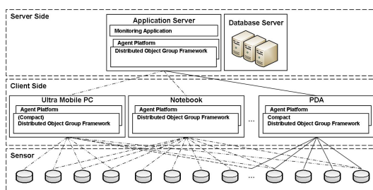
(그림 6) 헬스케어 상황정보 서비스 플랫폼의 시스템 환경
