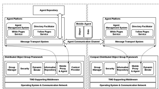
(그림 2) 헬스케어 상황정보 서비스 플랫폼
