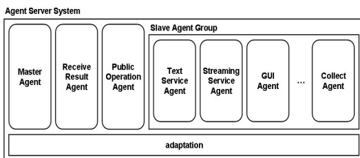
(그림 3) 멀티 에이전트 서버 시스템의 에이전트
