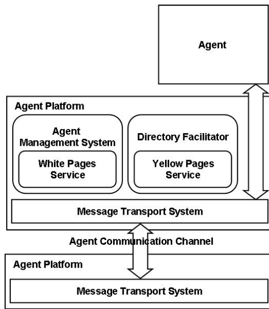
(그림 1) FIPA Agent Platform
