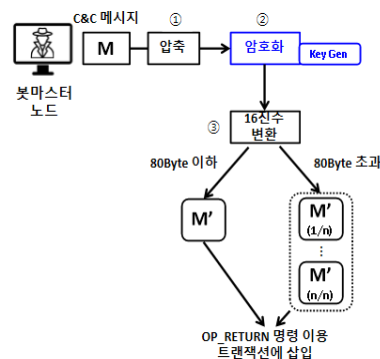
(그림 5) 암호화된 C&C 메시지 생성 절차 (Figure 5) Generation of Encrypted C&C Message
