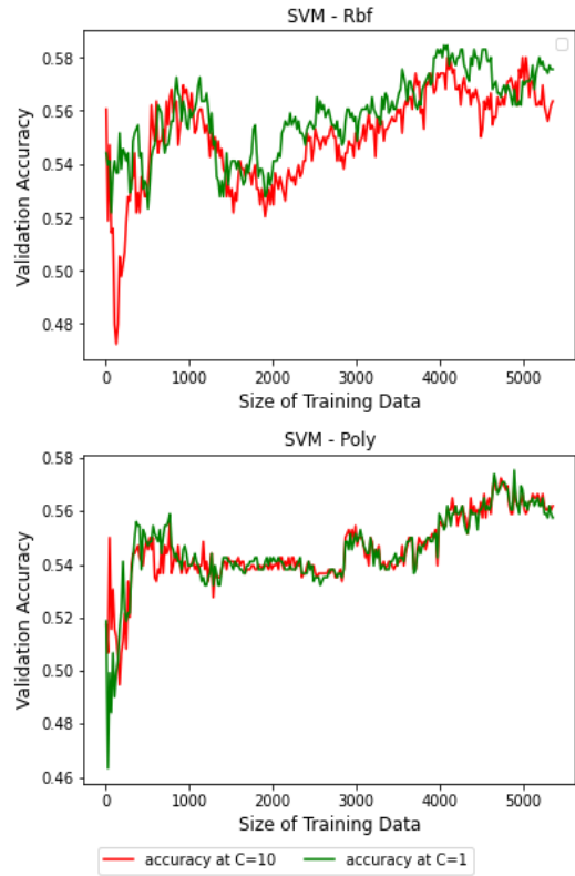
(그림 4) 훈련 데이터 크기에 따른 검증 정확도(Support Vector Machine)
