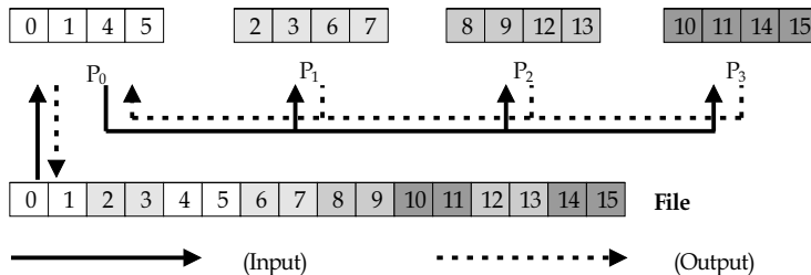
(그림 4) 순차 입출력과 MPI 전송 함수를 이용한 방식 (Figure 4) Sequential I/O and MPI functions
